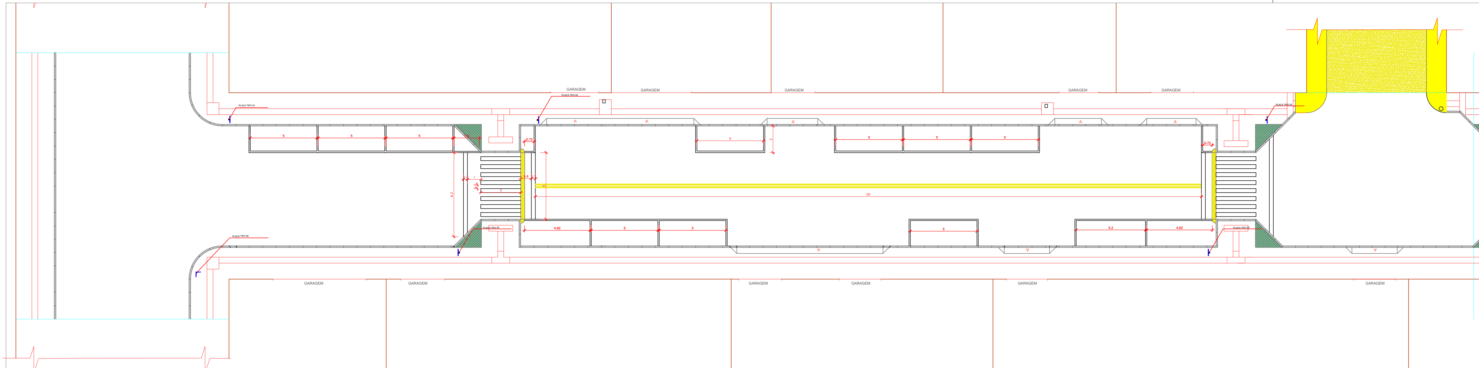
PLANTA DE SINALIZAÇÃO ESC 1/150
