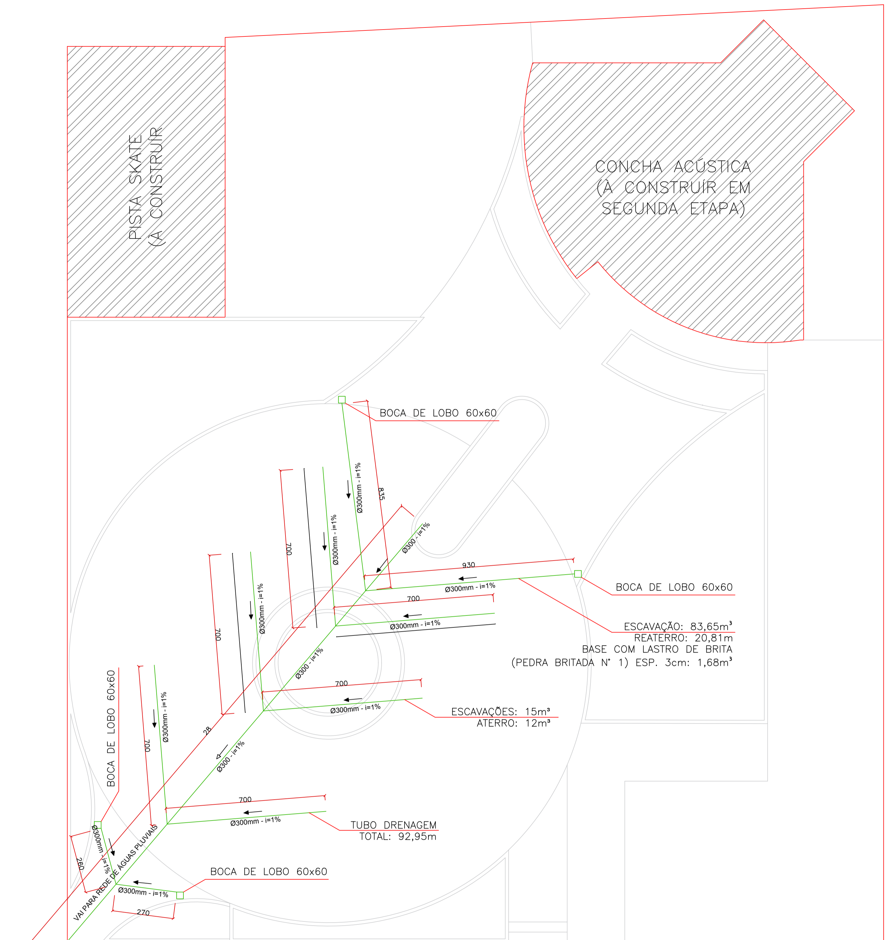
PLANTA DE DRENAGEM TERRENO MUNICIPAL ESCALA 1:100
