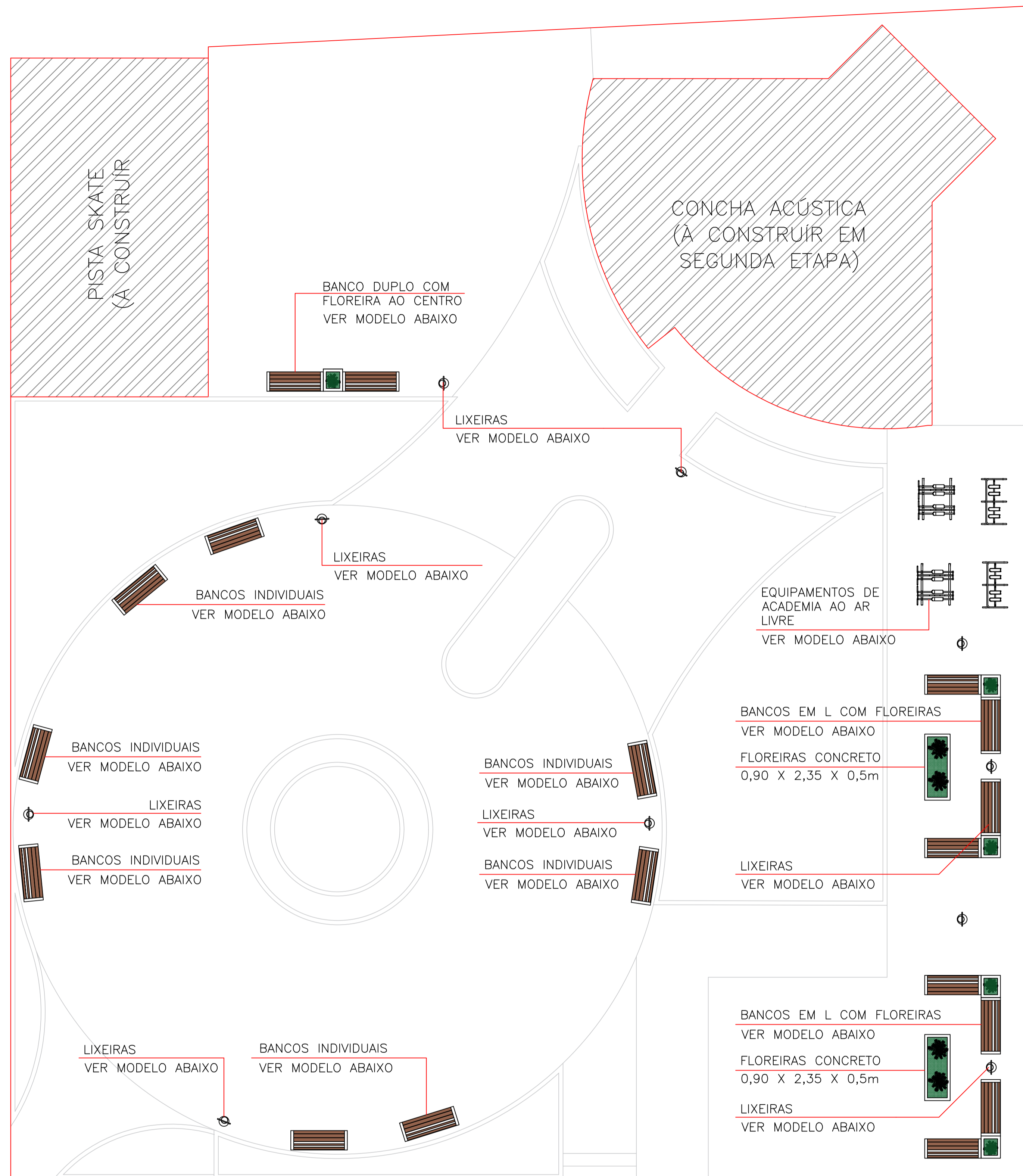
PLANTA DE MOBILIÁRIO TERRENO MUNICIPAL ESCALA 1:100
